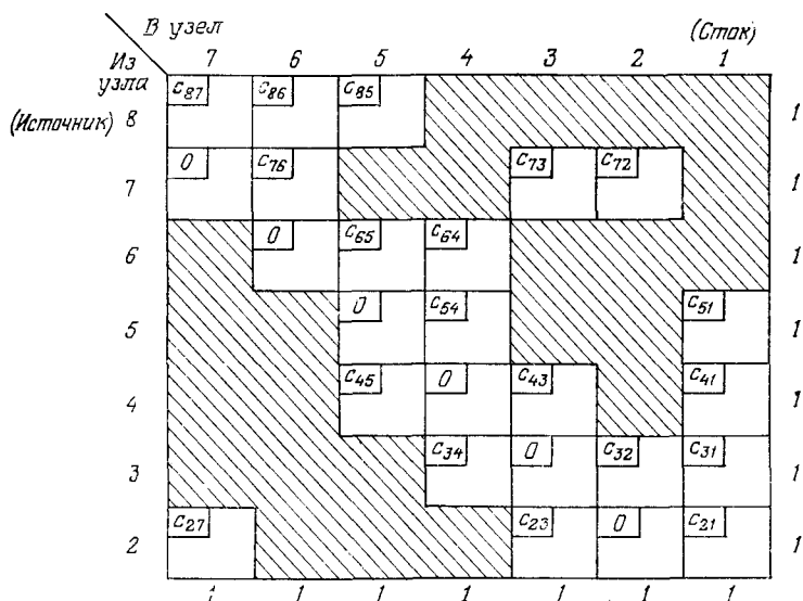
Р и с. 6.9. Матричное представление условий задачи о кратчайшем пути.
