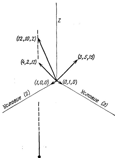
Р и с. 3.7. Геометрическое представление целевой функции в пространстве условий.
