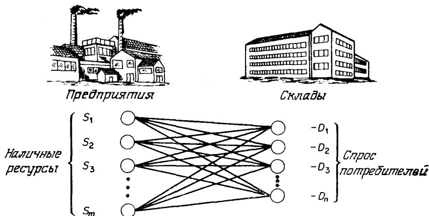
Р и с. 6.1. Сеть транспортной задачи.
