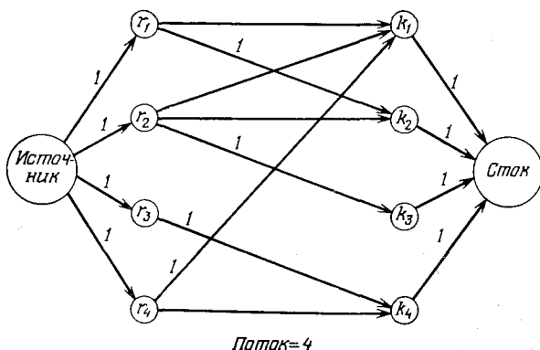
Р и с. 1.18. Окончательное решение.
