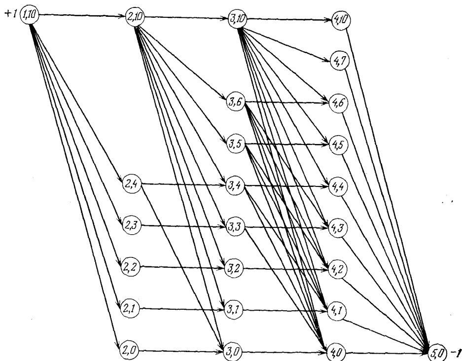
Рис. 6.11. Сеть, отображающая задачу компании «Новые просторы».
