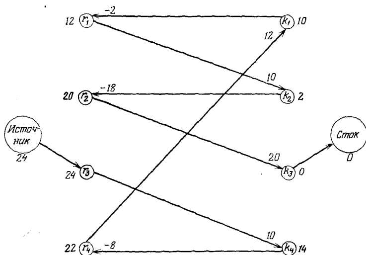
Р и с. I.20. Кратчайший маршрут.
