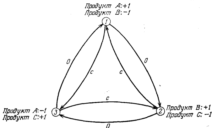
Р и с. 6.22. Многопродуктовая сеть.
