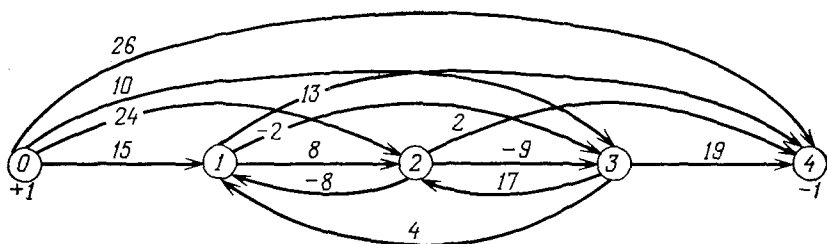
Р и с. I.24. Сеть, соответствующая методу решения задачи о назначениях размерности 4 \times 4 .
