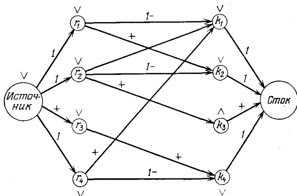
Р и с. 1.17. Измененная сеть.
